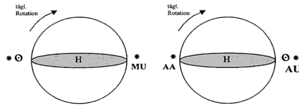
Abb. 39a: H: Horizont MA: Morgenaufgang MU: Morgenuntergang
